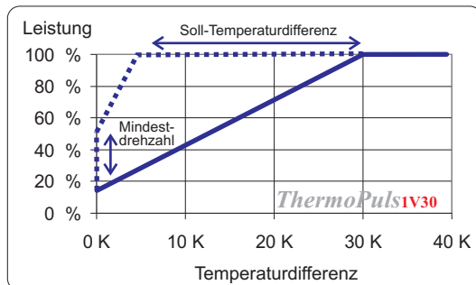
Kennlinie
